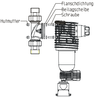
Abb. 3: Seitenansicht BOXER® RD
