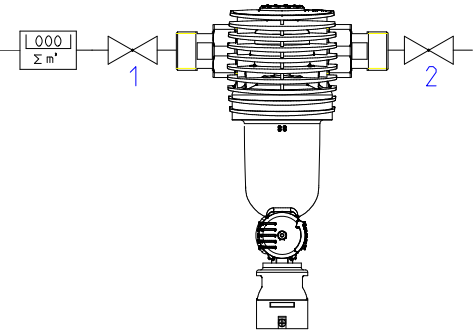
Abb. 2: Installationszeichnung BOXER® R Vorderansicht
