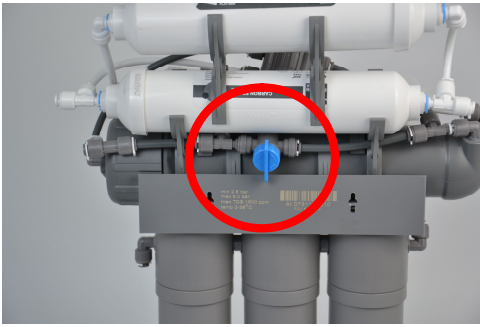
Geschlossenes Spülventil NEO 5-7
