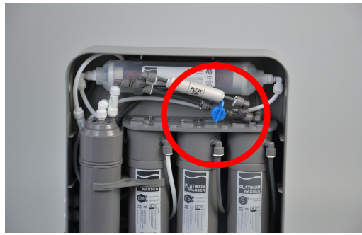
Geschlossenes Spülventil NEO-7 Box
